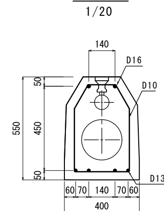
配筋図
