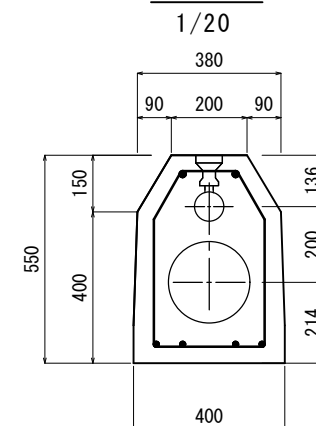
断面図
