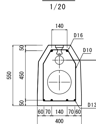
配筋図
