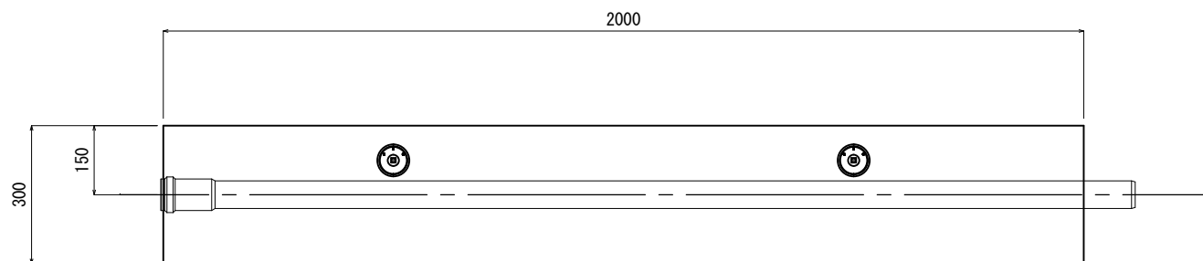
側面図
