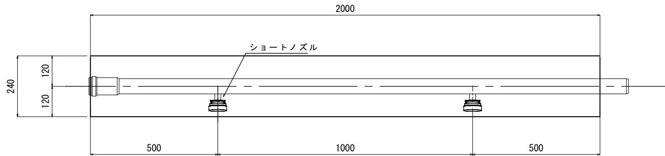
平面図
