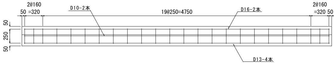
平面図
