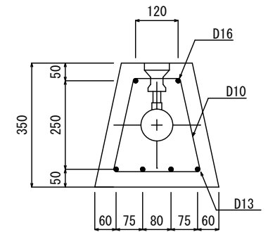
配筋図
