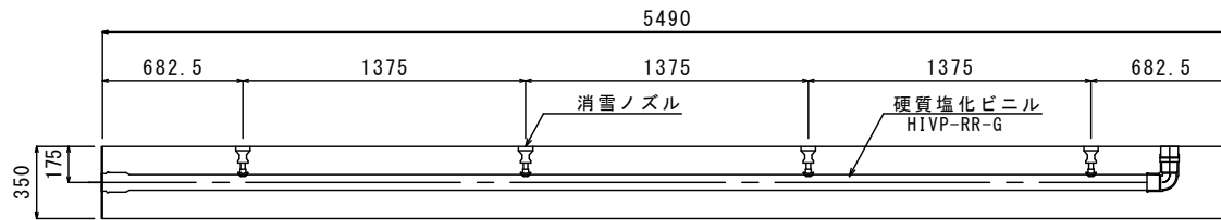
平面図
