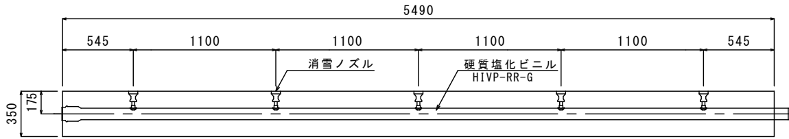
平面図
