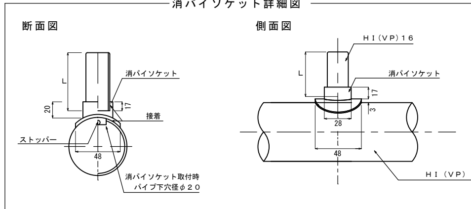
消パイソケット詳細図
